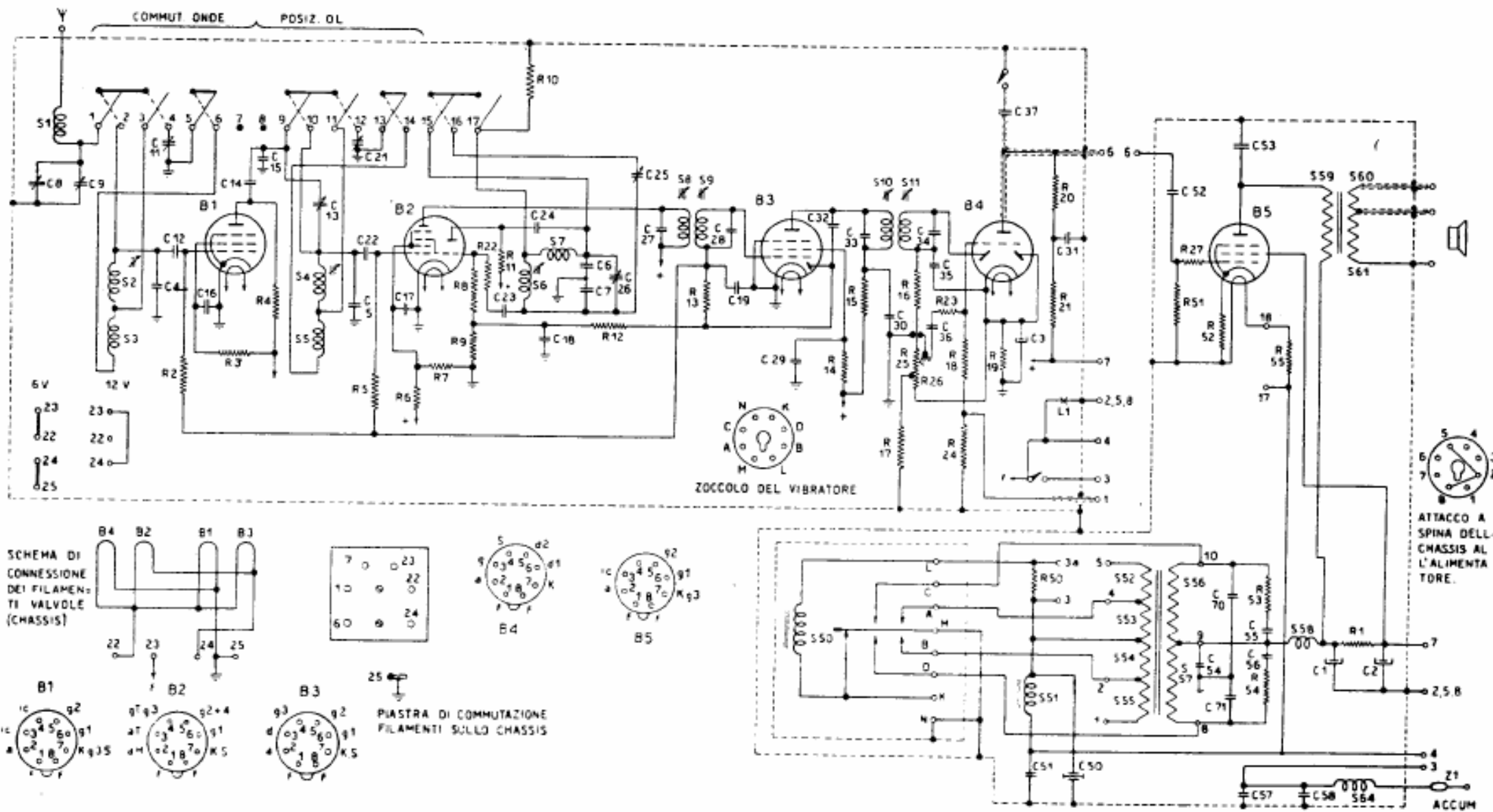
PHILIPS RADIO - Autoradio Mod. NL 524/V12. Consiste di una unità ricevente per onde lunghe e medie, e di una unità ricevente separata per onde corte. Nelle sei gamme OC funziona a doppia conversione di frequenza con l'aggiunta di una valvola. Consumo 2,8 A a 12 V. (V. valori a parte).
